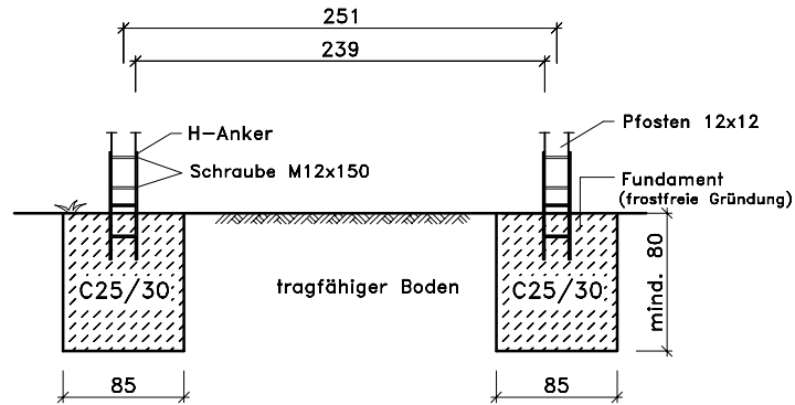
Schnitt A-A
