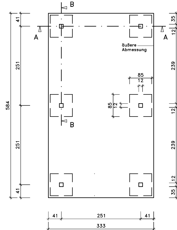
Grundriß
