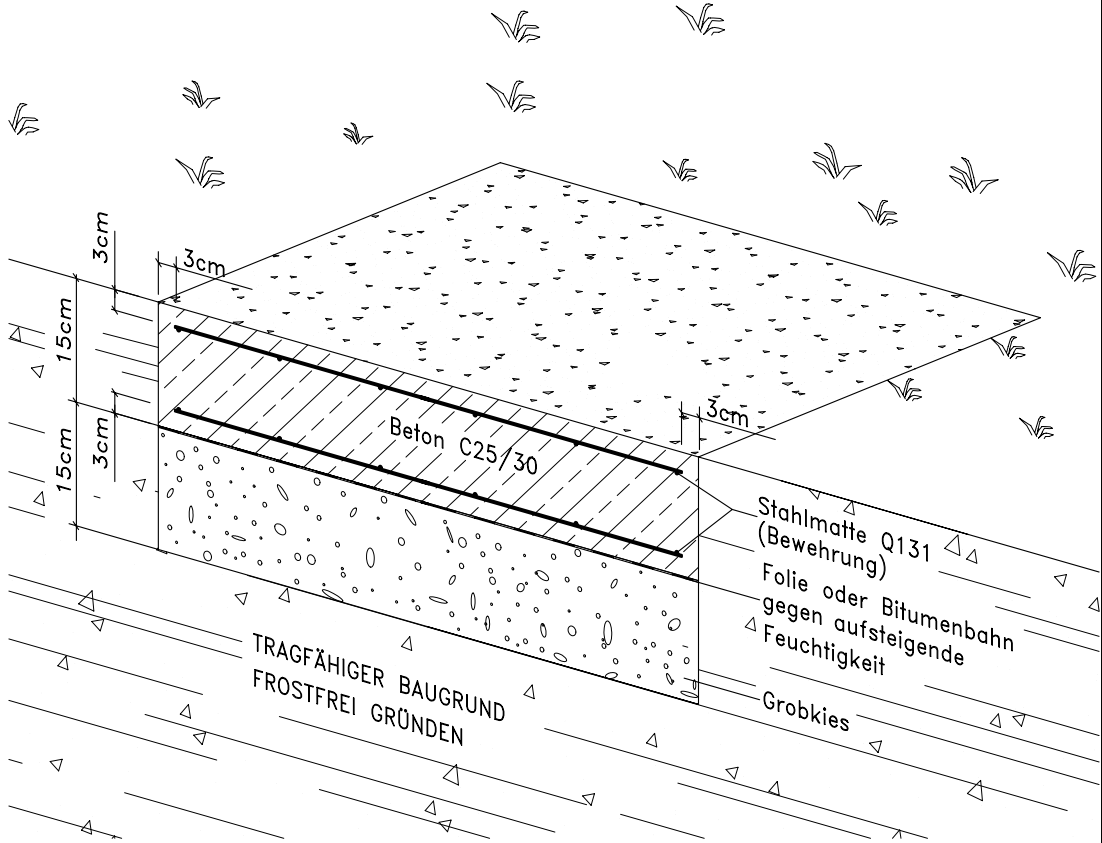
Schnitt A-A
