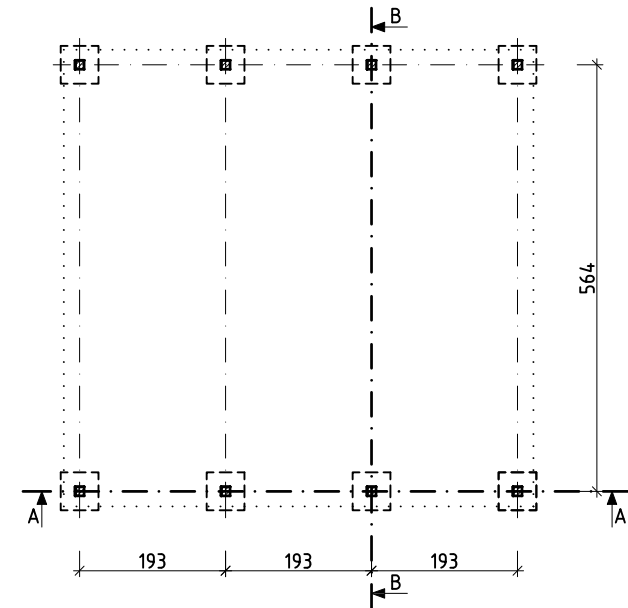
Grundriss M 1:100
