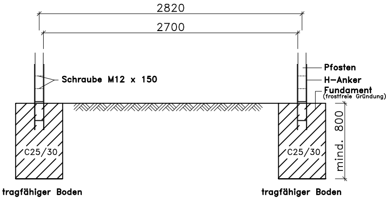
Schnitt B-B
