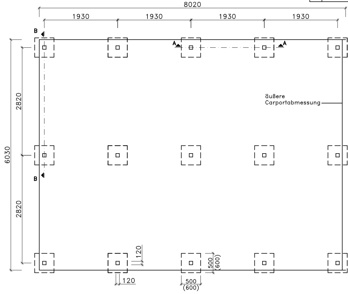
Grundriß
